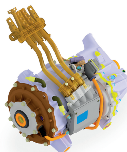
AUTOMOTIVE Hybridgetriebe mit E-Motor
